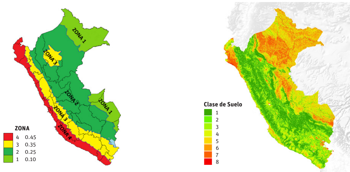
Figura 2-2 Zonificación de la amenaza sísmica y efectos de amplificación dinámica del suelo
